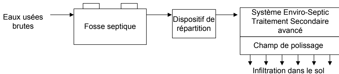
Fig. 2.2 : Système de traitement secondaire avancé
