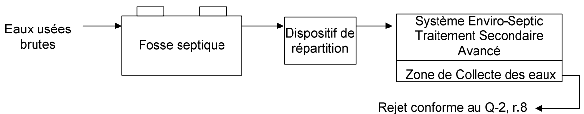
Fig. 3.2 : Système de traitement secondaire avancé
