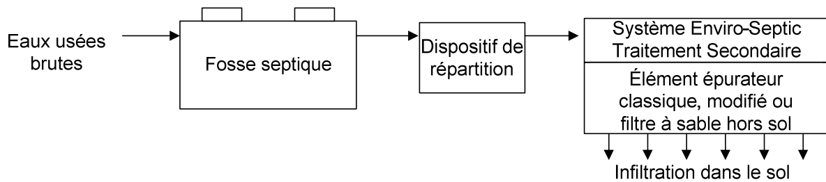
Fig. 2.1 : Système de traitement secondaire
