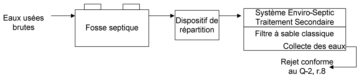
Fig. 3.1 : Système de traitement secondaire
